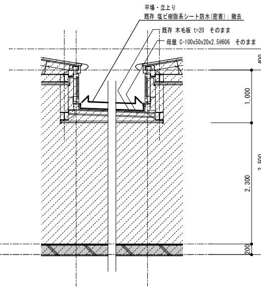
D-D' 部 現況断面図 S=1/50
