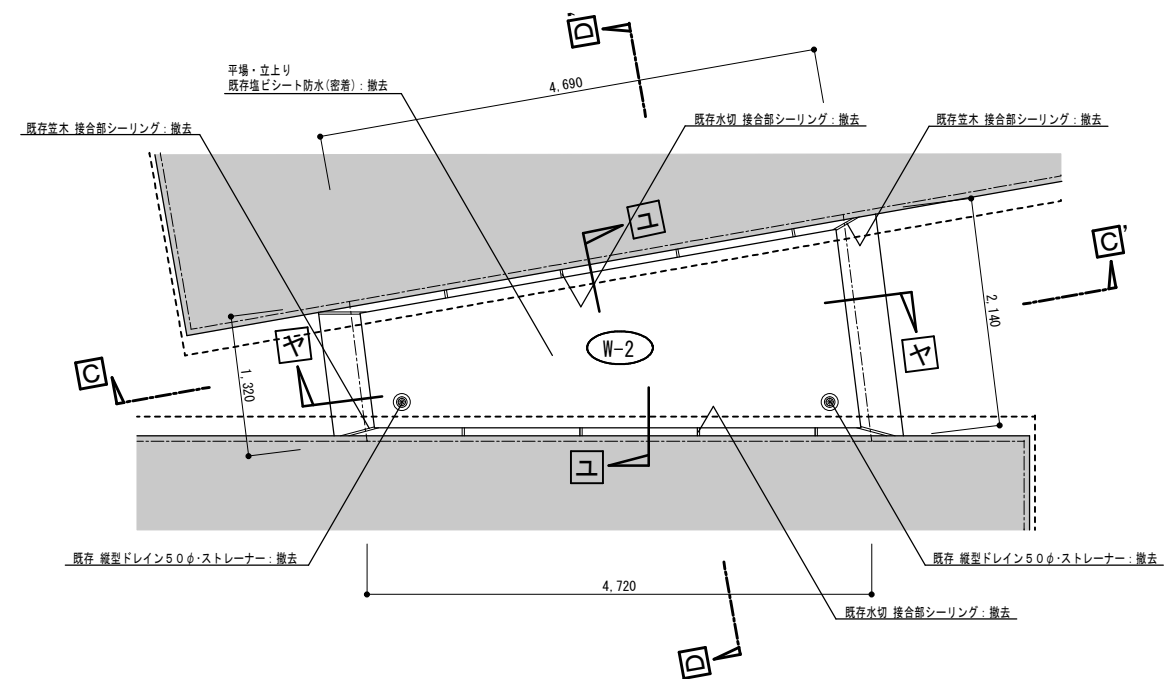
現 況 渡り廊下棟 屋根伏図 S=1/50
