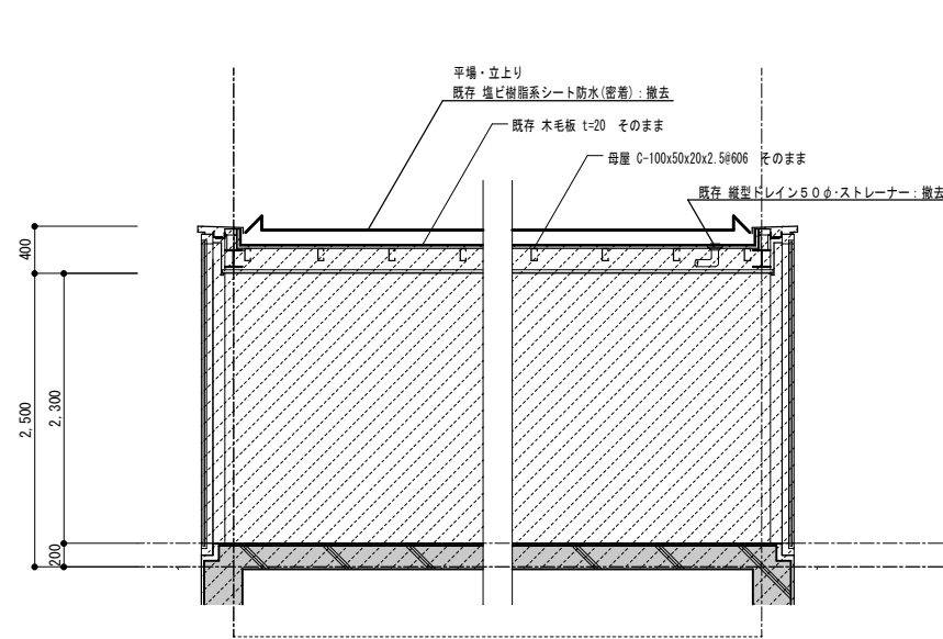
C-C' 部 現況断面図 S=1/50
