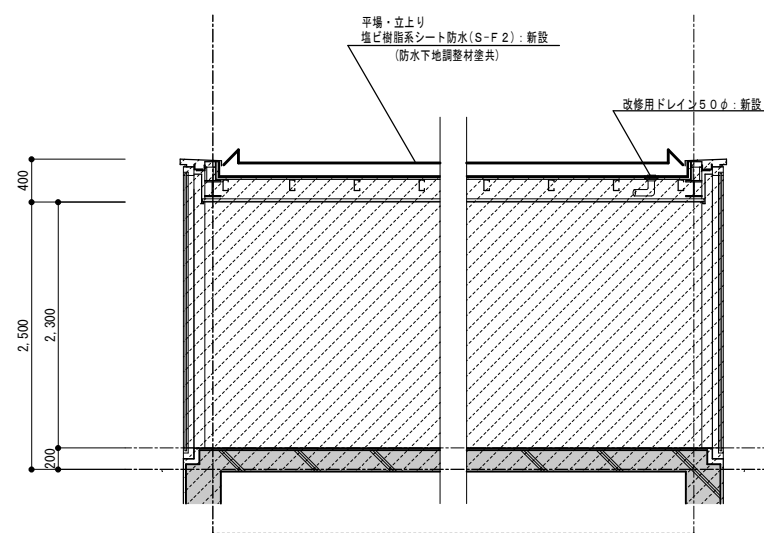
C-C' 部 改修後断面図 S=1/50
