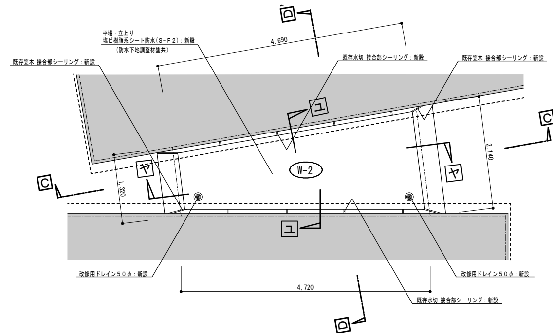
改修後 渡り廊下棟 屋根伏図 S=1/50
