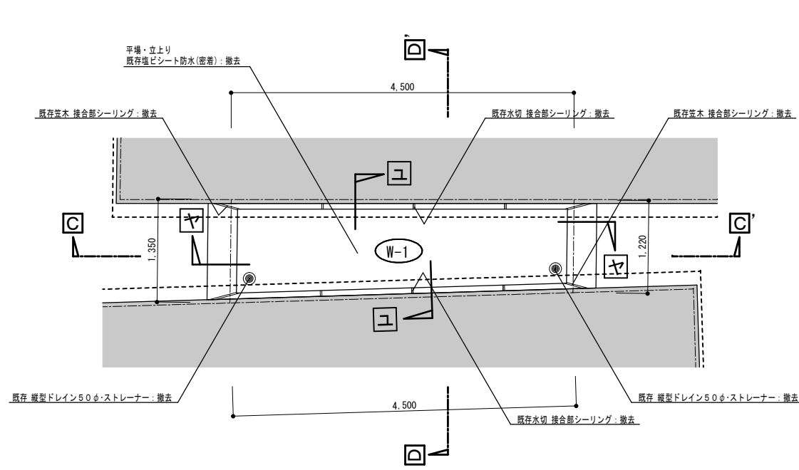
現 況 渡り廊下棟 屋根伏図 S=1/50
