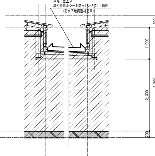
D-D' 部 改修後断面図 S=1/50
