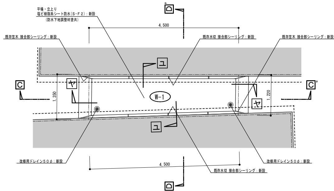
改修後 渡り廊下棟 屋根伏図 S=1/50
